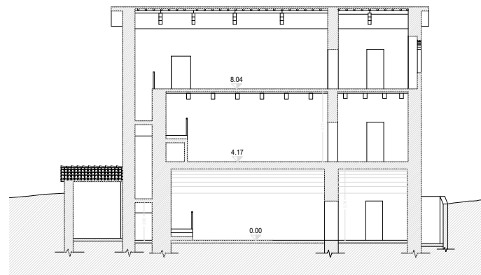
SEZIONE B-B
