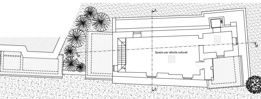
PIANO SECONDO
