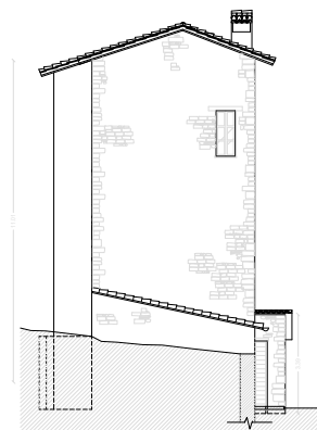
PROSPETTO OVEST
