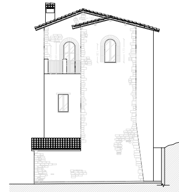
PROSPETTO EST
