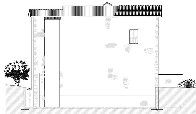
PROSPETTO NORD
